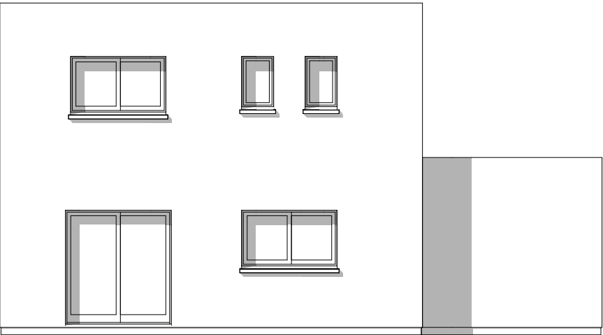
Façade arrière
