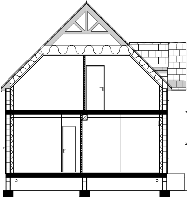
Coupe
