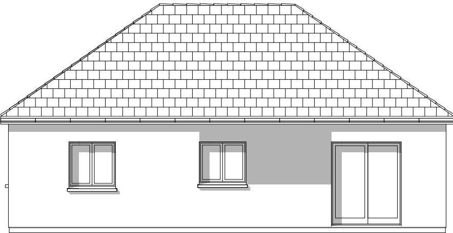
Façade arrière
