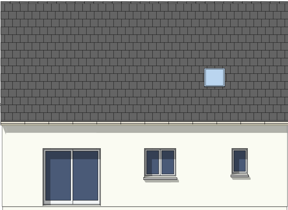
Façade arrière
