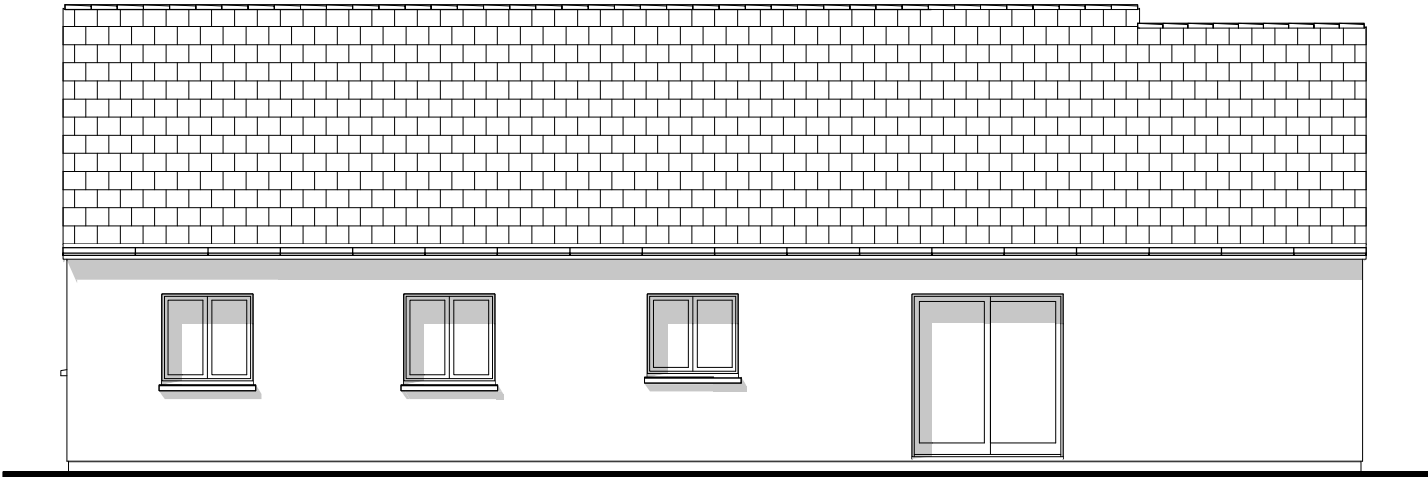
Façade arrière
